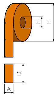
SOBRE EXTERIOR TERMOSELLABLE TAMAÑO DE LA BOBINA
