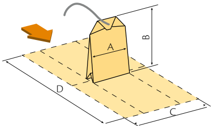
TAMAÑO DEL SAQUITO
